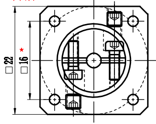
输入端Input
